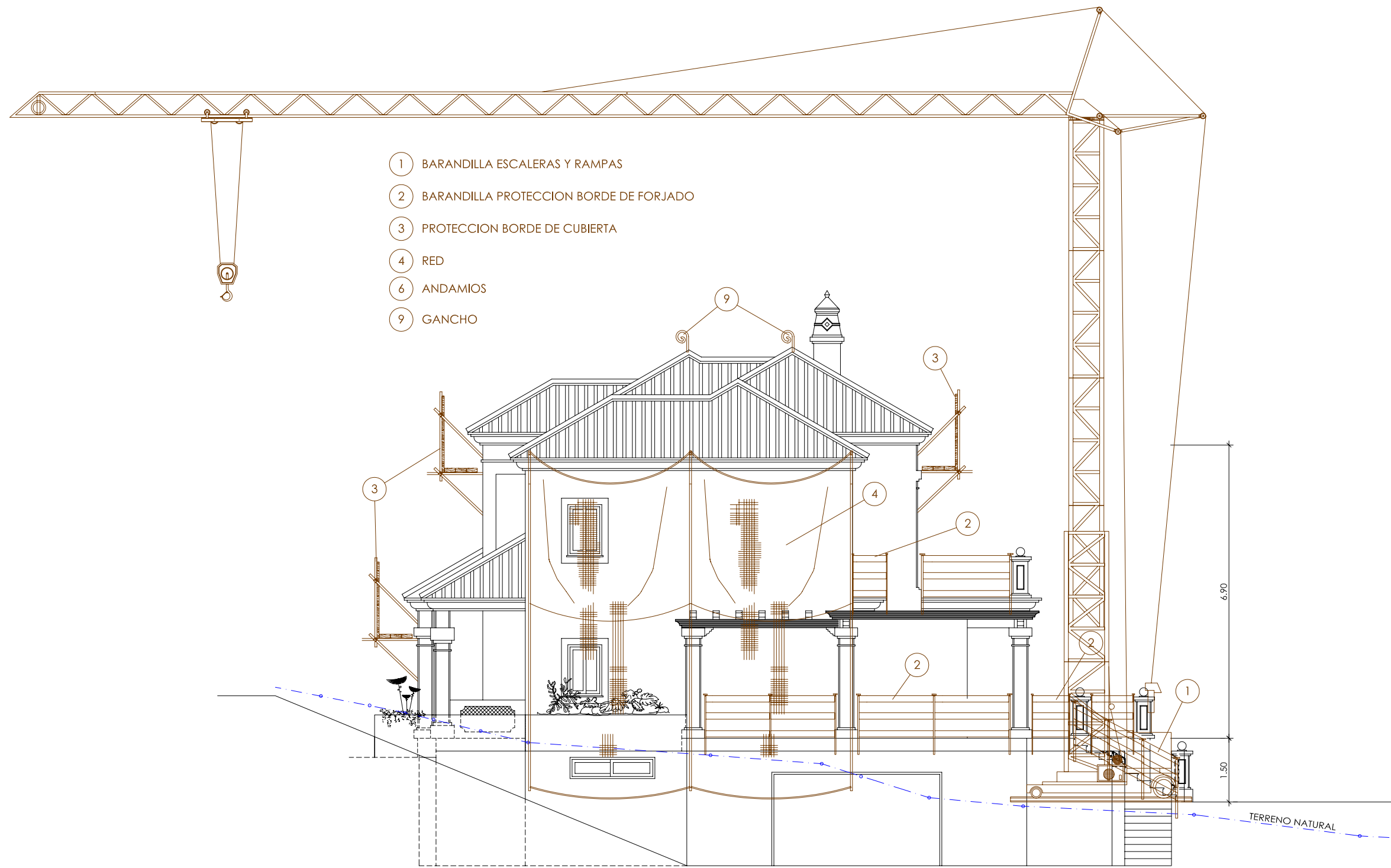
ALZADO LATERAL DERECHO
